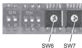
Рис. 15 Настройка адреса Modbus
