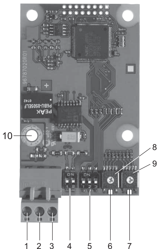
Рис. 13 Модуль CIM 2XX Modbus
