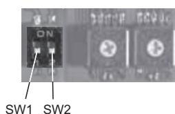
Рис. 12 Включение и выключение согласующих резисторов
