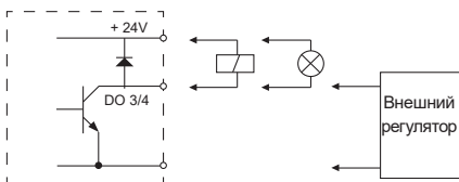
Рис. 41 Пример настраиваемых цифровых входов или выходов
