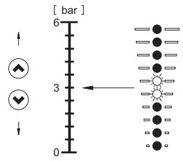
Նկար 15 3 մ սահմանված նշանակություն, կառավարում ըստ ճնշումների տարբերության
