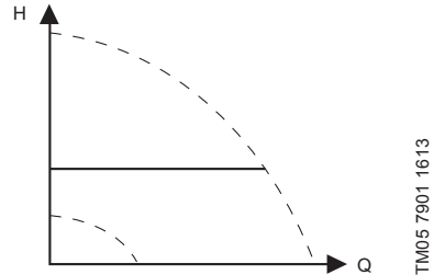
Նկար 25 «Մշտական ճնշում»
