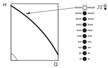
Նկար 17 Առավելագույն բնութագրի ռեժիմ
