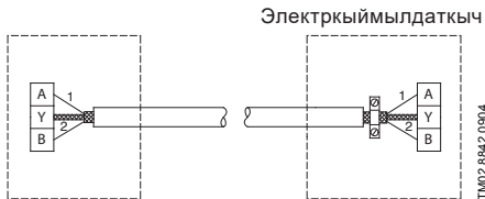
Сүрөт 12 2 жылкалуу экрандаштырылган кабелди туташтыруу
