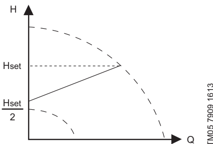
Նկար 23 «Համամասնական ճնշում»
