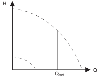
Рис. 33 «Постоянный расход»
