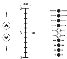
15-сүр. Белгиленген маани 3 м, басымдын олку-солкулугун боюнча башкаруу
