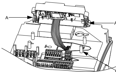
60-сурет Пластик қақпақты орналастыру
