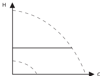
25-сурет «Тұрақты қысым»
